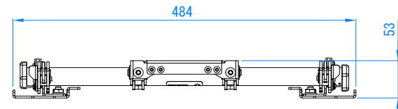
400mmアダプター(付属品)取付時
