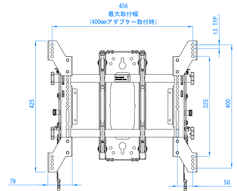
400mmアダプター(付属品)取付時
