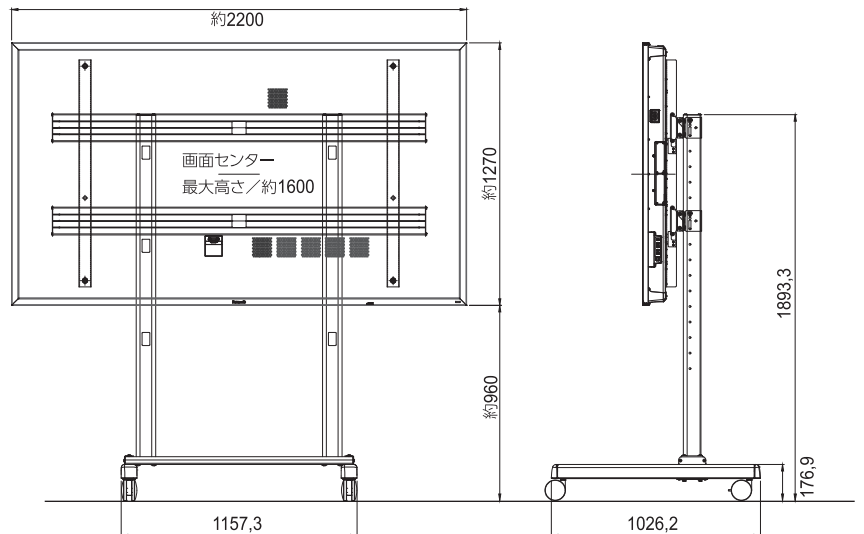
基本設置図 / 98型ディスプレイ取付時 [単位: mm]
