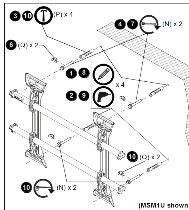
【図-2-b】 コンクリート壁面取付け例
